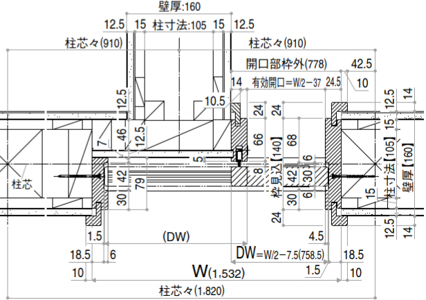
●横断面図 枠見込140
