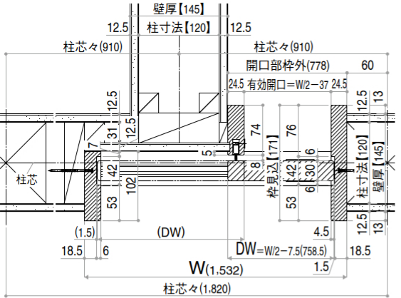
●横断面図 枠見込171
