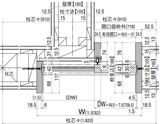
●横断面図 枠見込186
