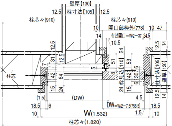
●横断面図 枠見込110
