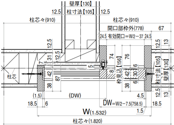
●横断面図 枠見込156
