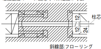
埋込敷居(アルミ)使用時の床貼込み寸法
