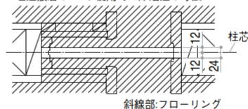
埋込敷居(アルミ)使用時の床貼込み寸法
