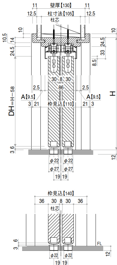
基本寸法表
