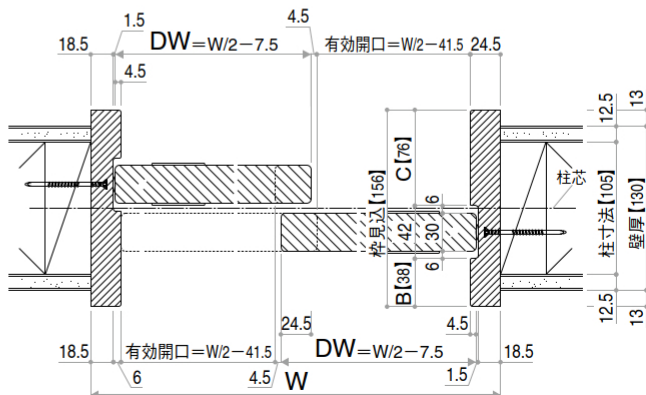
●横断面図
