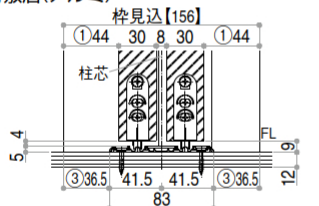
●横断面図 引違い戸(4枚建)
