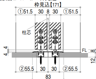
●横断面図 引違い戸(2枚建)
