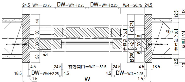
●横断面図 引違い戸(4枚建)
