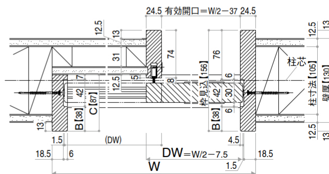
●横断面図
