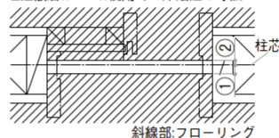
斜線部:フローリング
