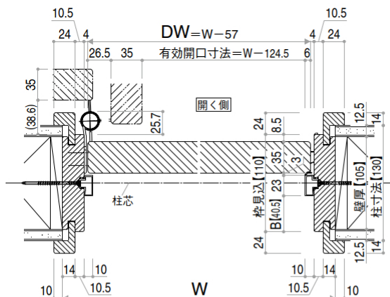
●横断面図 (片開きドア・トイレドア・ペットドア)
