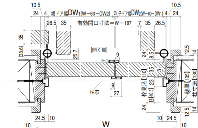
●横断面図 (親子ドア)
