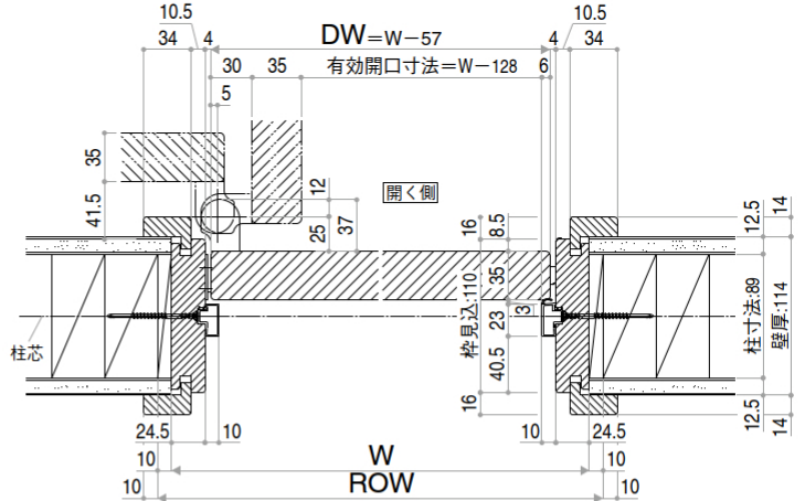
●横断面図 (片開きドア・トイレドア・ペットドア)
