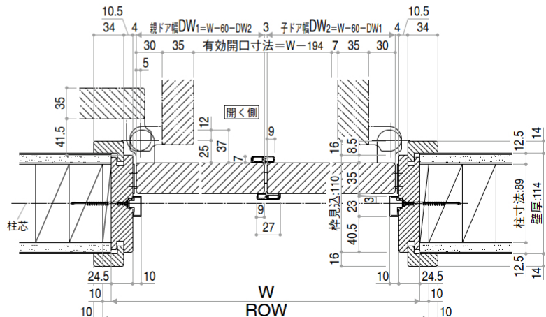
●横断面図 (親子ドア)
