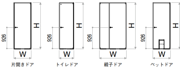
基本寸法 (mm) 片開き・トイレ・ベット 親子 W呼称 064 073 075 077 082 087 118 W(DW) 648(591) 733(676) 752(695) 778(721) 823(766) 878(821) 1,188(721/407) 有効開口 520 605 624 650 695 750 994 H呼称 20 H(DH) 2,033(1,989)
