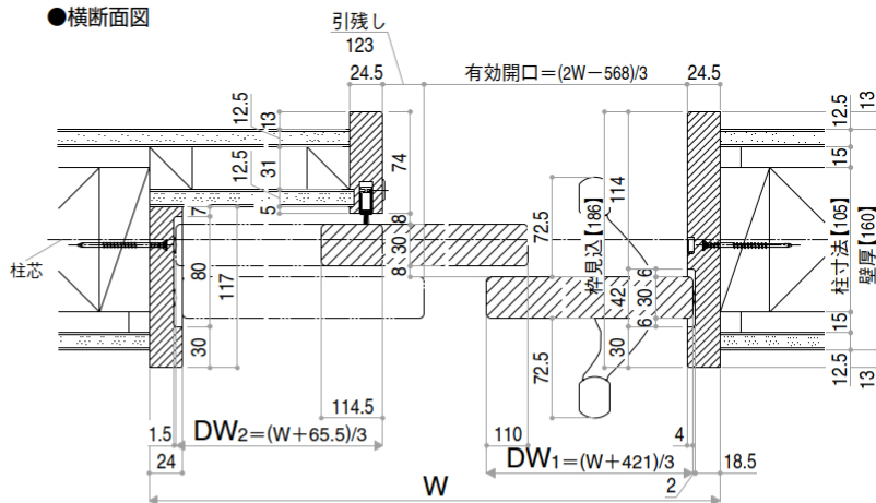
●横断面図
