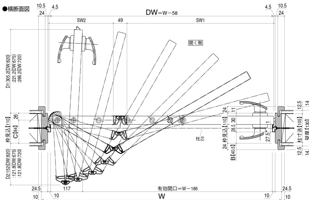
SW1、SW2寸法算出公式
