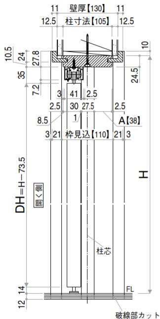
【床後貼】 ・薄沓摺(シート)
