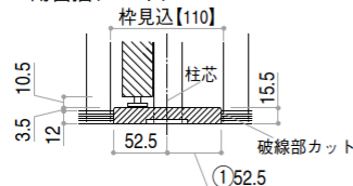
【床後貼】 ・薄沓摺(シート)
