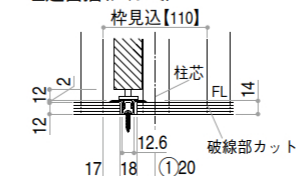
【床先貼】※取付位置：柱芯基準 ・埋込沓摺(アルミ)
