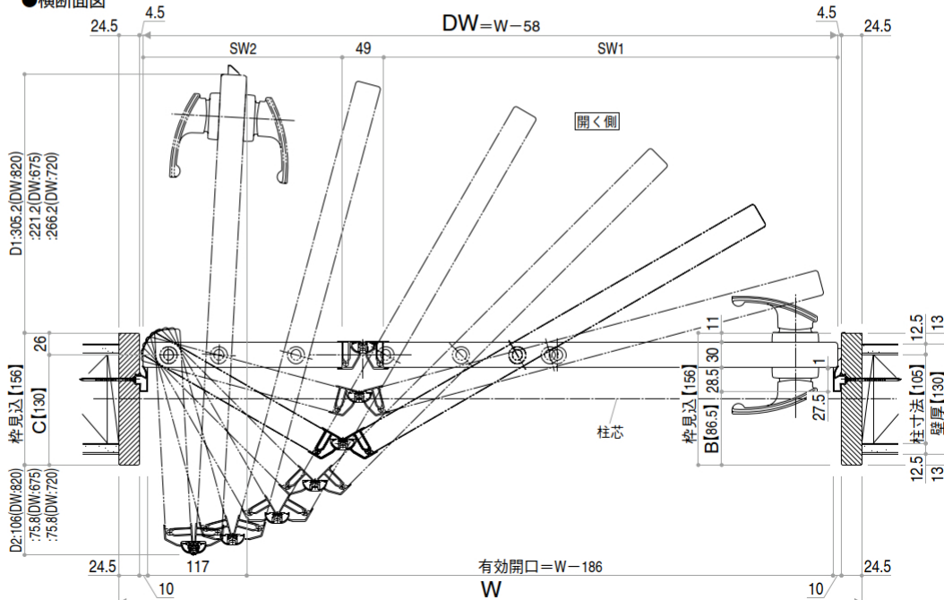
●横断面図
